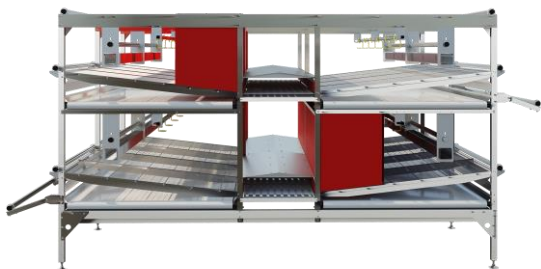
СИСТЕМА БЕЗКЛЕТОЧНОГО СОДЕРДАНИЯ ДЛЯ Кур-Несушек Baltika-4
