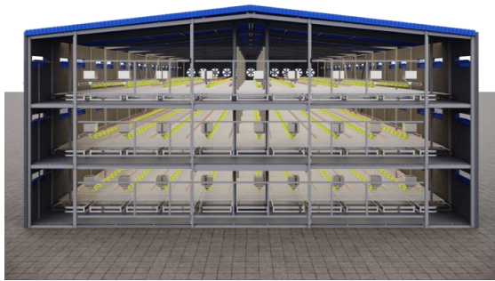
СИСТЕМА ВЫРАЩИВАНИЯ БРОйлЕРА НА СЕТЧАТЫХ ПОЛАХ MaxGrow
